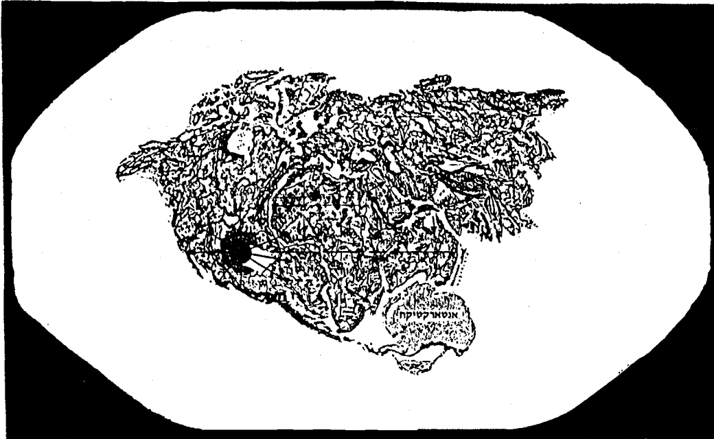
יבשת בראשית לדעת הגיאולוגים
