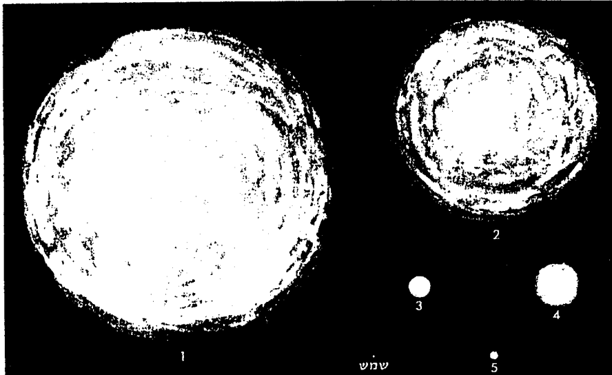
ענקים ועל-ענקים בהשוואה לשמש 1. \alpha בענון (Auriga), קטרו כ-3/2 מיליארד ק"מ; 2. \beta בפאסוס; 3. קאפלה [העור'] \alpha בענון; 4. ארקטורוס \alpha ברוטה הסוורים (Bootes); 5. \gamma בברנור (Cygnus). קוטר השמש - 1.4 מיליון ק"מ
