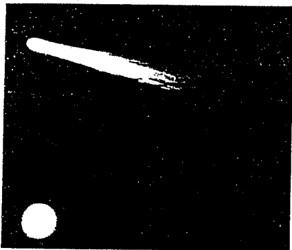
כוכב השביט הלי בביקורו בשנת ז'תר"ע (1910). מצד שמאל למטה כוכב השחר נוגה (ונס).
