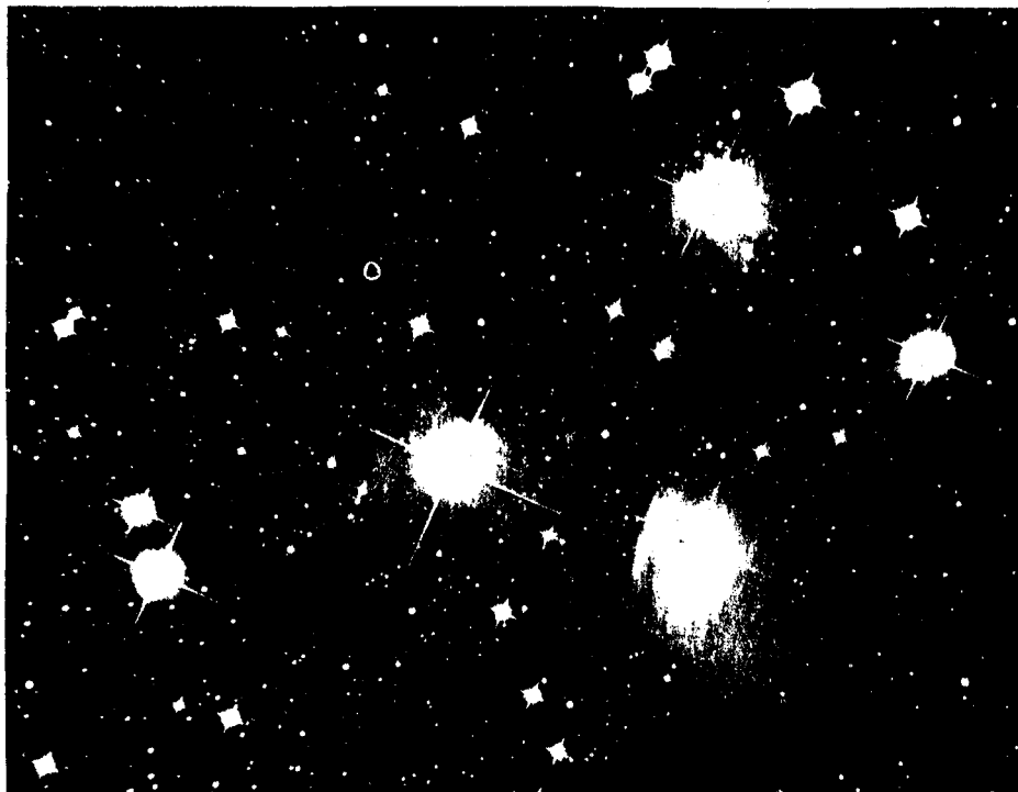
צביר הכוכבים כימה (פליאדות) כפי שנצפה בטלסקופ החלל ע"ש האבל (HUBBLE) וצולם במצלמות CCD מתוחכמת המחוברת לטלסקופ
