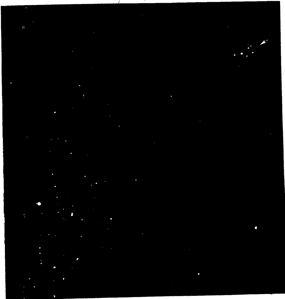
צביר הכוכבים כימה (פליאדות) נמצא בפינה הימנית העליונה (מסומן בחץ) כפי שנראה בעין רגילה
